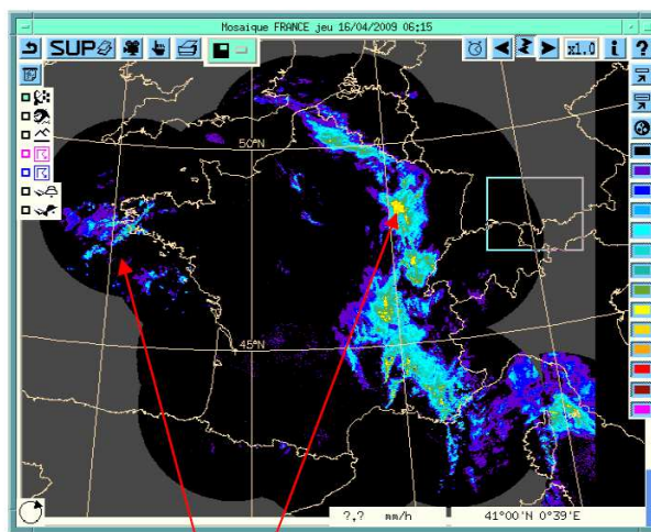
2. Exemple de front pluvio-instable avec traîne peu active : averses faibles loin à l'arrière
